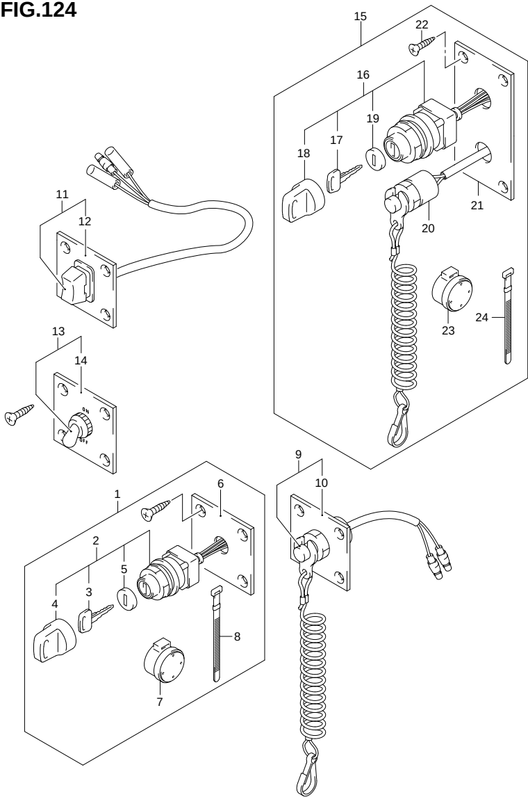
DF100 115 E01 012_124 OPT:SWITCH
