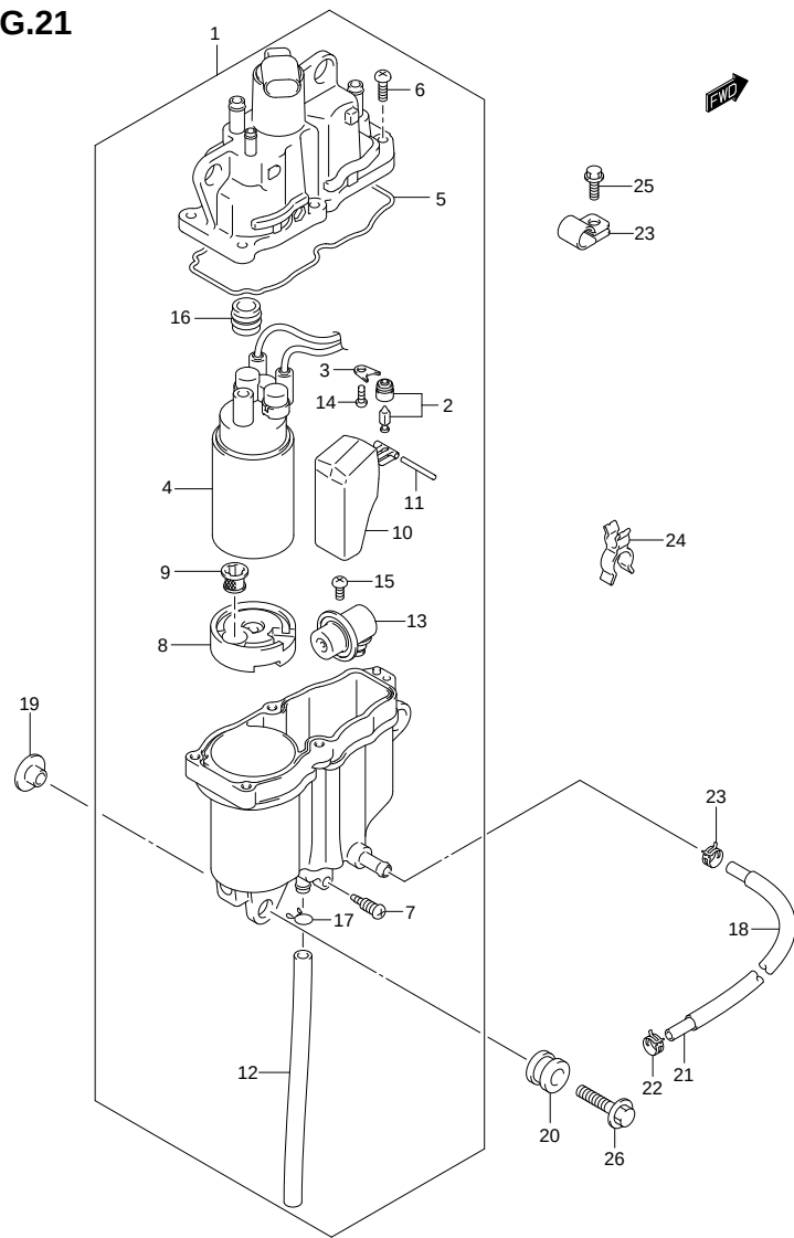
FIG. 21 (1-C-14) FUEL VAPOR SEPARATOR (DF115T E1)
