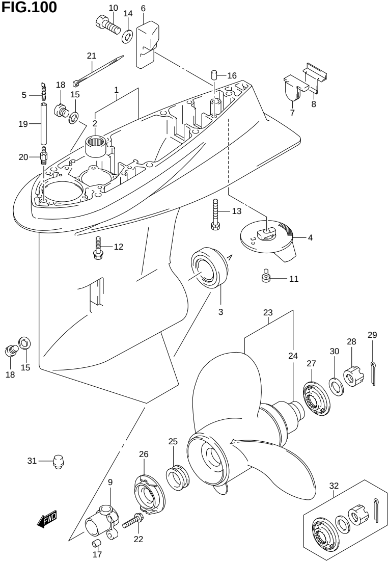
DF100 115 E01 012_100 GEAR CASE
