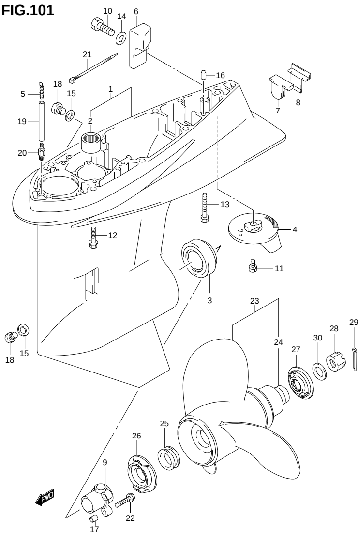
DF100 115 E01 012_101 GEAR CASE
