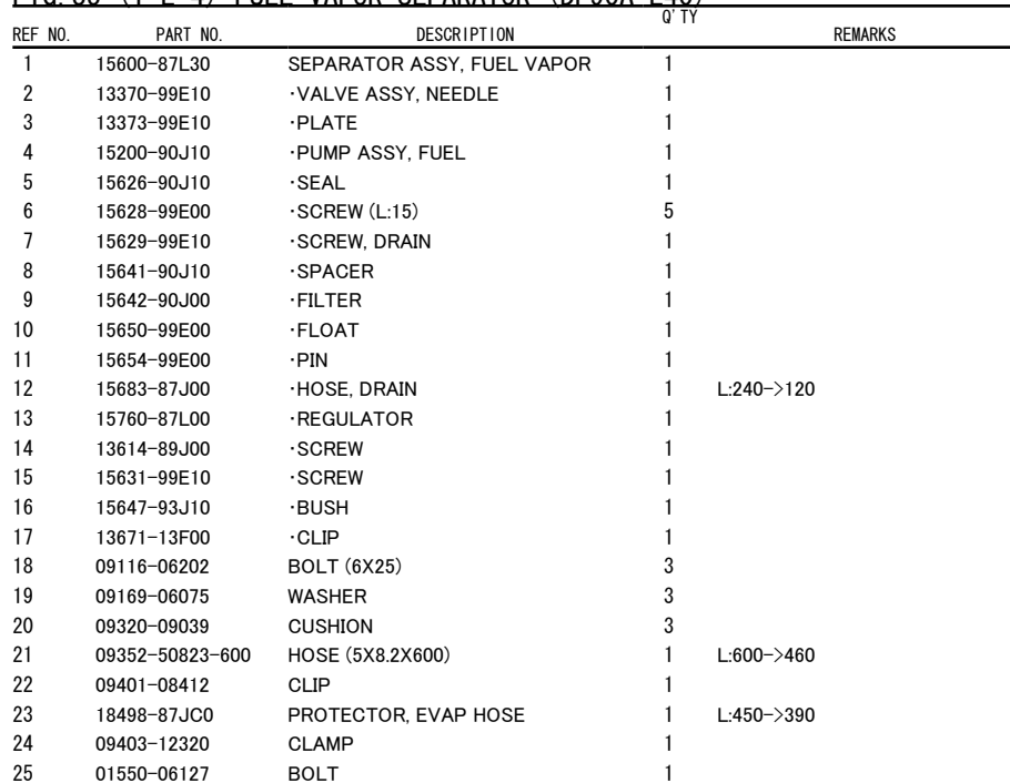
FIG. 35 (1-E-4) FUEL VAPOR SEPARATOR (DF90A E40)
