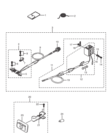
Fig. 15 OPTIONAL PARTS (3) ACCESSORIES オプションパーツ (3) アクセサリ
