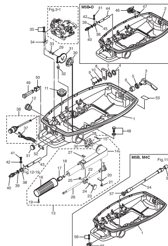
Fig. 9 BOTTOM COWL • TILLER HANDLE ボトムカウル・ティラハンドル
