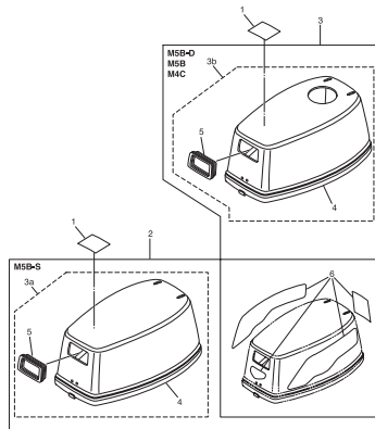
Fig. 10 TOP COWL トップカウル
