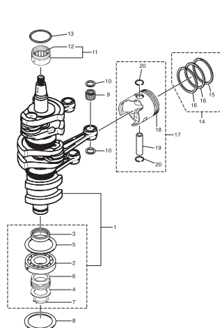
PISTON・CRANK SHAFT ピストン・クランクシャフト
