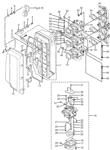
INTAKE SILENCER・CARBURETOR インテークサイレンサ・キャブレタ
