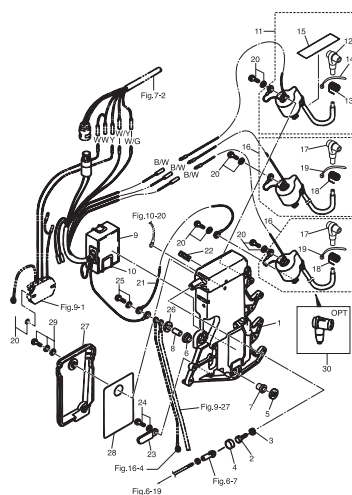
エレクトリックパーツ (C.D. ユニット)
