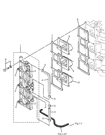
Fig. 3 INTAKE MANIFOLD・REED VALVE インテークマニホールド・リードバルブ
