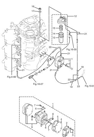
FUEL LINE フュエルライン
