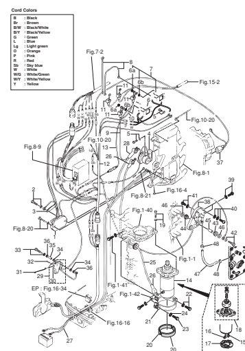
エレクトリックパーツ（スタータモータ）
