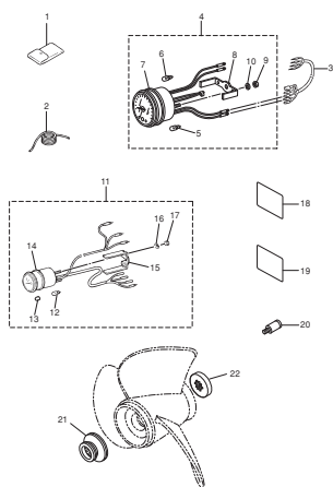
Fig. 24 OPTIONAL PARTS (3) オプションパーツ (3)
