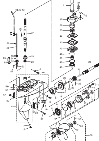
GEAR CASE ギヤケース
