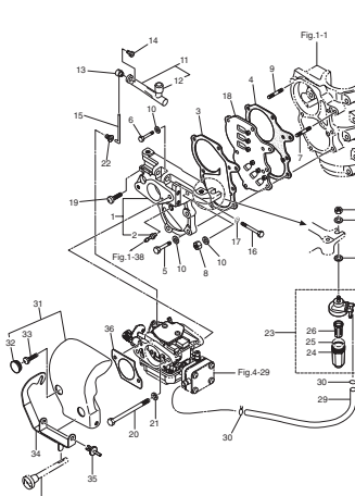
インタークマニホールド
