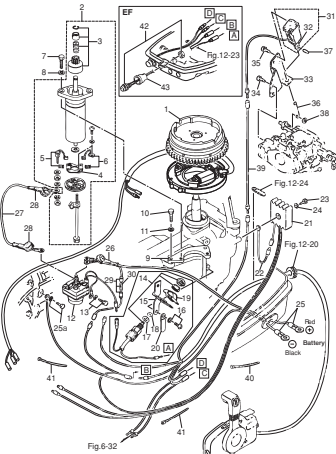
ELECTRIC STARTER (EF・EP MODEL) トレクトリックスターター(EF・EPモデル)
