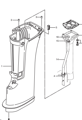
DRIVE SHAFT HOUSING ドライブシャフトハウジング
