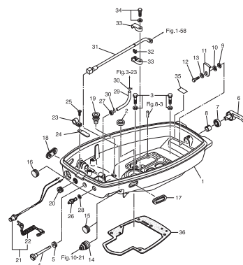
Fig. 12 BOTTOM COWL ボトムカウル
