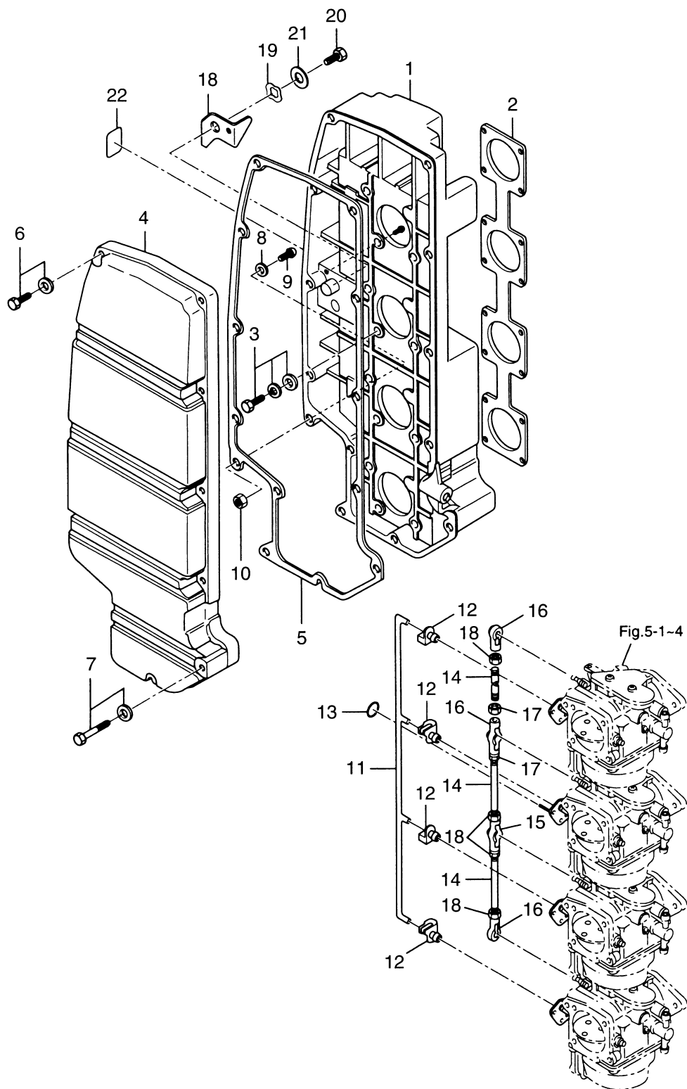
エアサイレンサ Fig. 4 AIR SILENCER
