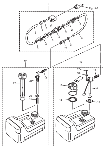
Fig.16 FUEL TANK フエルトンク
